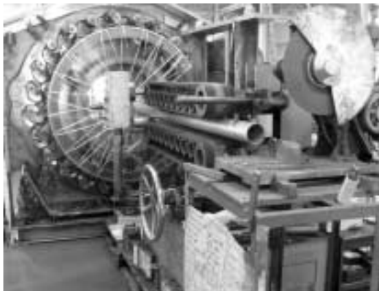
同社が保有する最大級の加工機。直径25号のホースに編み上げ加工を施せる。主な用途先は石油プラントなど
